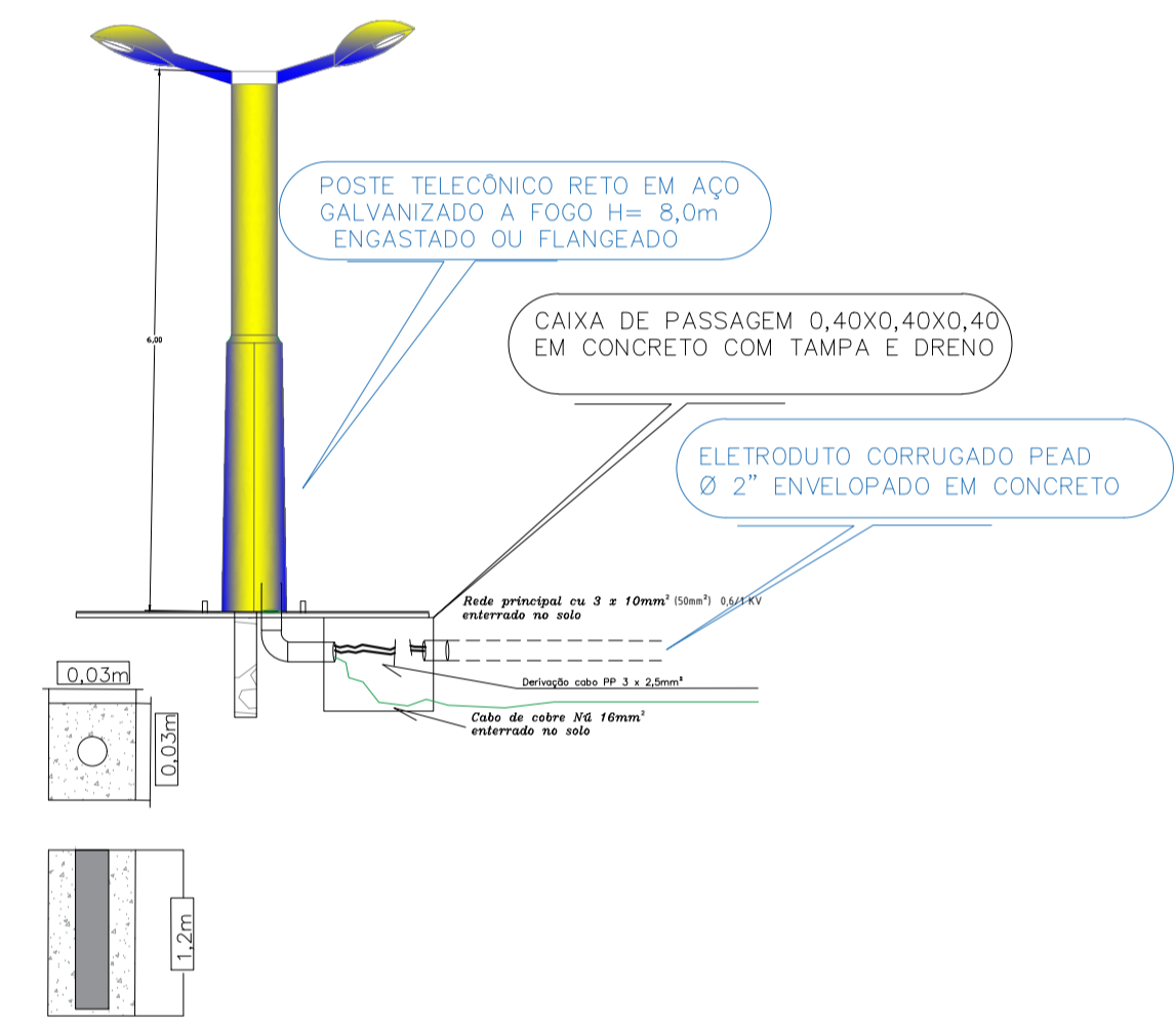
DETALHE DO POSTE DE ENTRADA S/ESCALA
