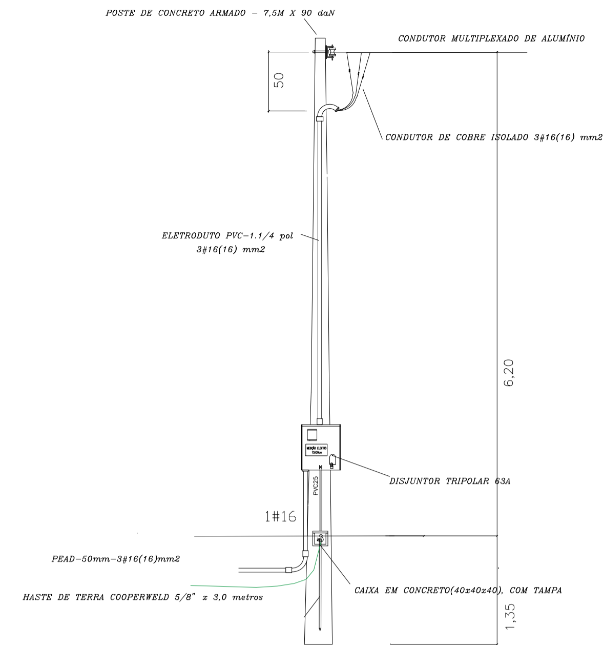
DETALHE DO POSTE DE ENTRADA S/ESCALA
