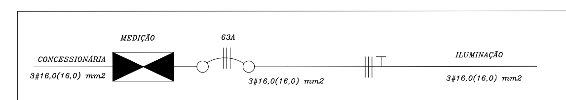
DIAGRAMA UNIFILAR - ILUMINAÇÃO PÚBLICA TRECHO - 2 AEREO
