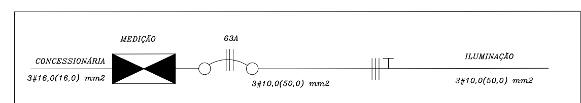
DIAGRAMA UNIFILAR - ILUMINAÇÃO PÚBLICA TRECHO - 1 SUBTERRANEO
