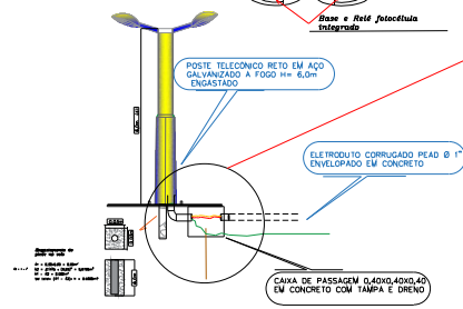
DETALHE DA LUMINÁRIA
