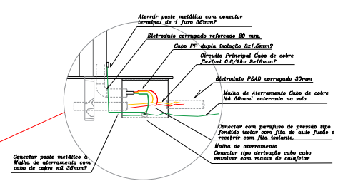
DETALHE CAIXA DE PASSAGEM 0,40X0,40X0,40 EM CONCRETO COM TAMPA E DRENO
