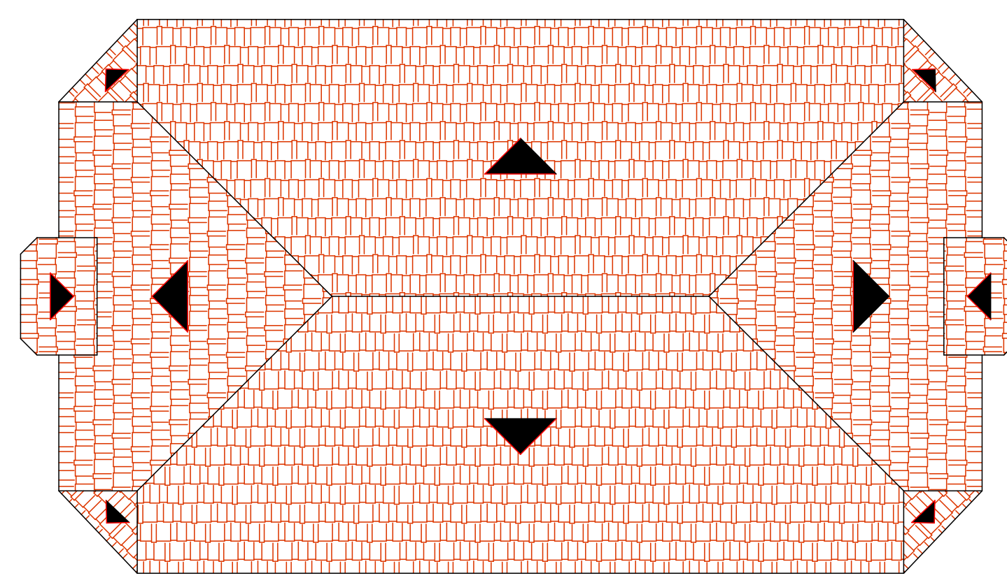
COBERTURA ESCALA 1:100
