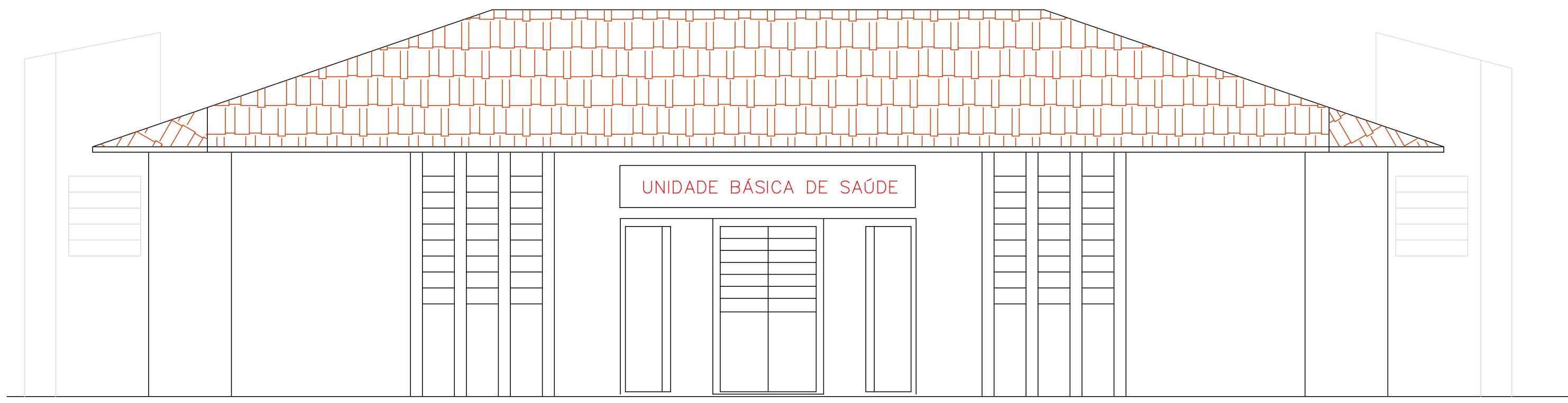
FACHADA ESCALA 1:50
