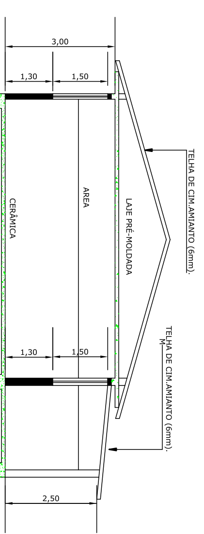
CORTE A - A'
